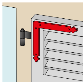
29PA9... Gegenwinkel Aluminium reversibel, Loch eckig, 34x4, Feston Contre-equerre aluminium réversible réglable, trous carrés, 34x4, feston Contro-T alluminio punta fiore 34 x e fori quadri
